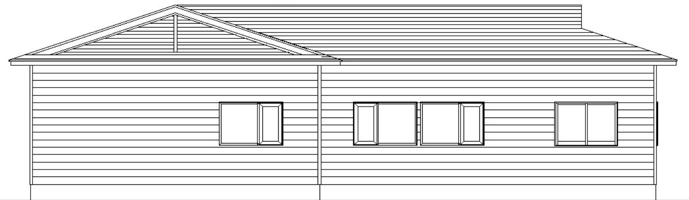
西面立面図
