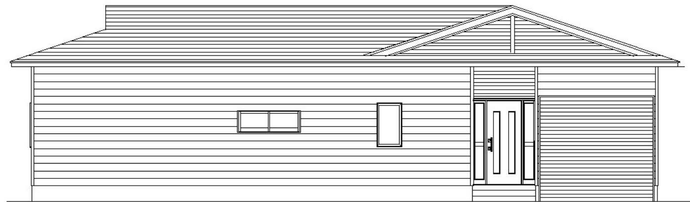
東面立面図
